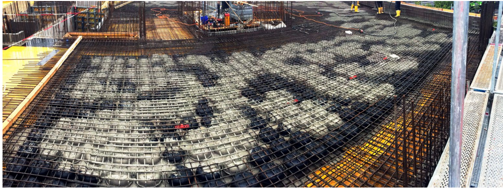
Eine werdende Cobiax SL Stahlbetondecke beim ersten Betoniervorgang.
